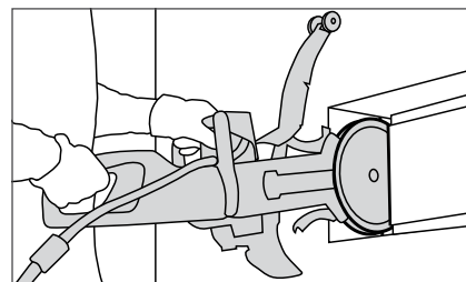
Menší úprava otvorů pro okna a dveře.
