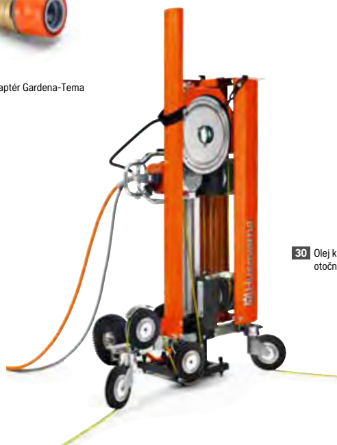
29 Dopravní vozík pro WS 220
