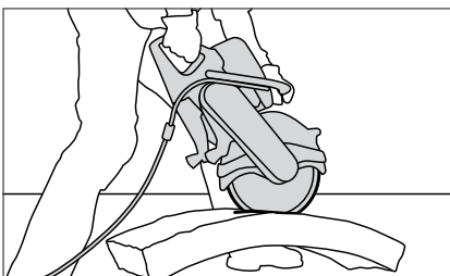
Řezání stavebních bloků, ohrubníků a zahradních dlaždic.
